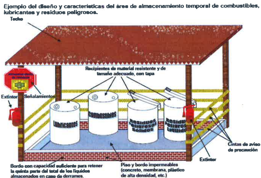
Figura 1. Prototipo de caseta para residuos peligrosos
