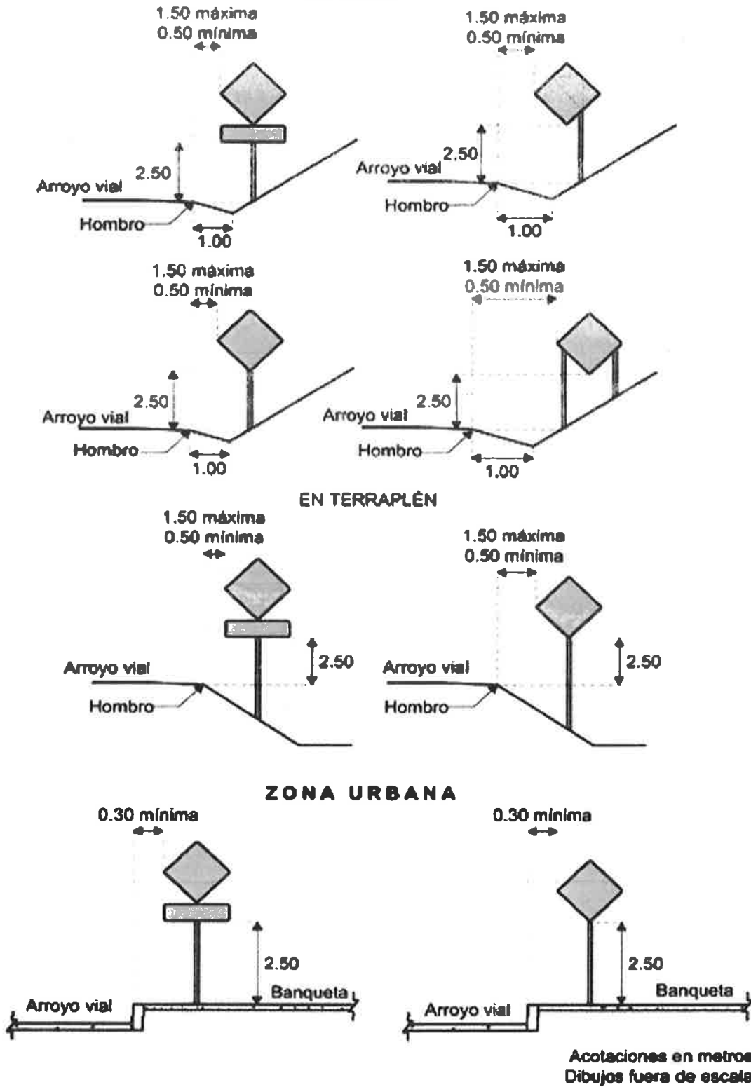
FIGURA 1.- Distancia lateral y altura de las señales preventivas.
