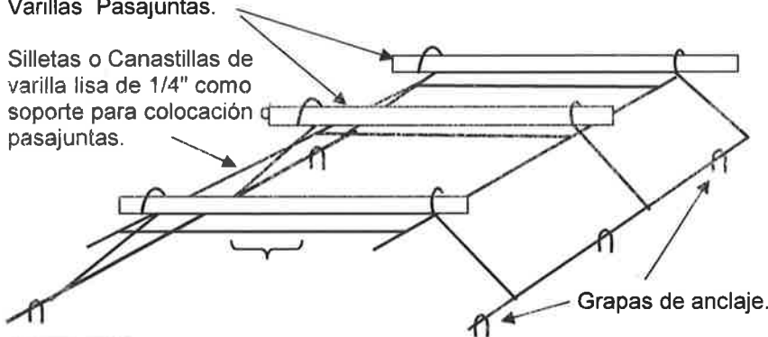
Fig. No.1 La sileta se deberá fijar a la sub base o base con grapas o clavos que garanticen que mantenga su posición durante el vaciado y compactación del concreto.
