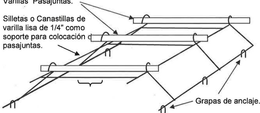
Fig. No.1 La silleta se deberá fijar a la sub base o base con grapas o clavos que garanticen que mantenga su posición durante el vaciado y compactación del concreto.
