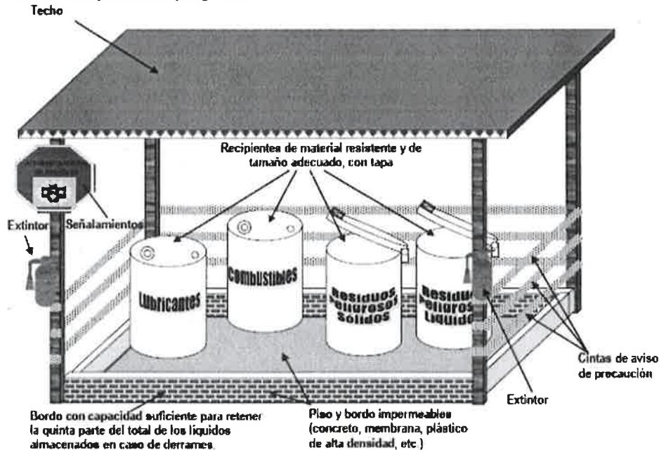
Figura 1. Prototipo de caseta para residuos peligrosos
