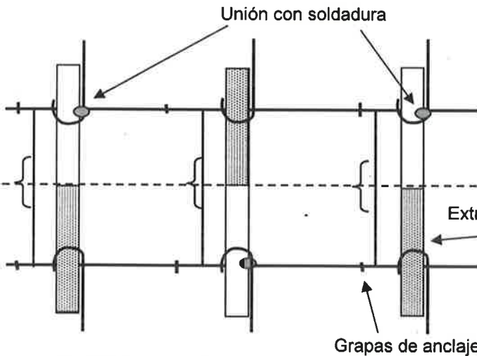
Fig. No.2 Vista en planta.
