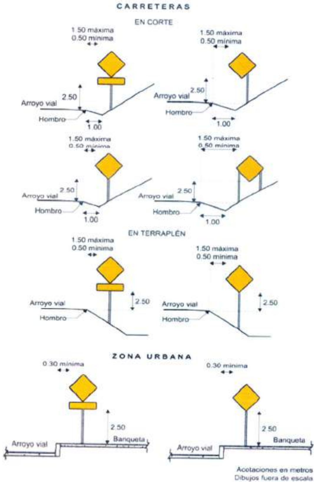
FIGURA 1.- Distancia lateral y altura de las señales preventivas.
