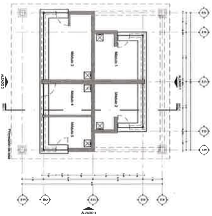
MOSCO COMERCIAL / PLANTA esc. 1/75
