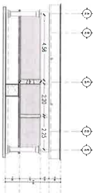
MOSCO COMERCIAL / ALZADO 2 esc. 1/75
