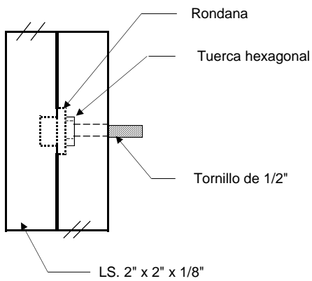
DETALLE "A"
