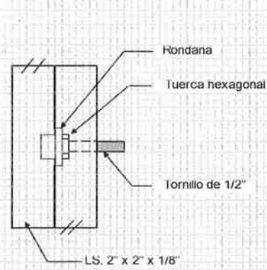
DETALLE "A"
