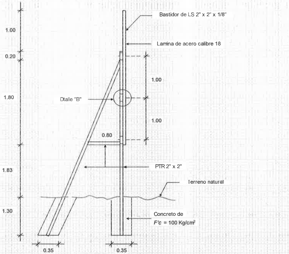
CORTE A-A'
